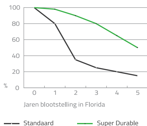
Blootstelling – glansbehoud
