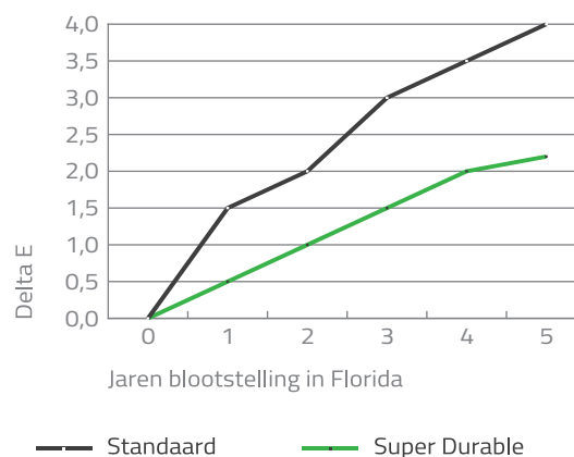
Blootstelling – kleurbehoud
